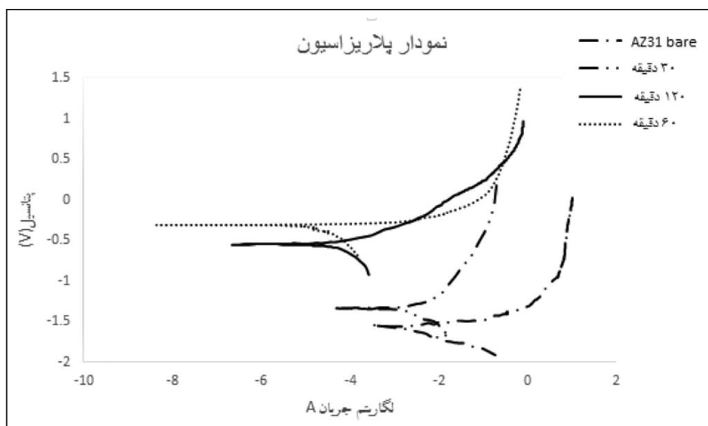
شکل ۶- منحنی پلاریزاسیون پوشش‌های نیکل فسفر الکترولس بر نمونه‌های زیرآیند، ۳۰ دقیقه، ۶۰ دقیقه و ۱۲۰ دقیقه آماده‌سازی شده در محلول \text{NaHCO}_3 ، در محلول ۰.۵٪ NaCl.
