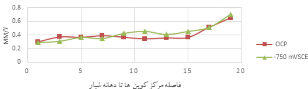
شکل ۱۰- مقایسه تغییرات وزنی در شرایط پتانسیل -۷۵۰ میلی‌ولت نسبت به اکترومد مرجع کالومل و پتانسیل مدار باز.
