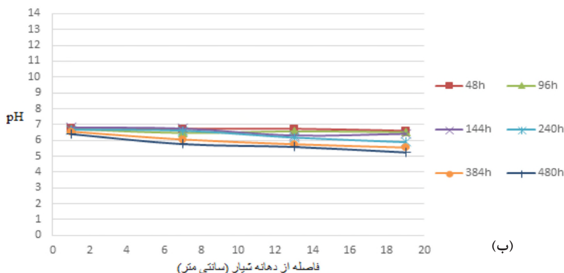
شکل ۸- (الف) نمودار تغییرات پتانسیل بر حسب فاصله از دهانه شیار در زیر پوشش جدا شده در شرایط پتانسیل مدار باز. (ب) نمودار تغییرات pH در زیر پوشش جدا شده بر حسب فاصله از دهانه شیار در شرایط پتانسیل مدار باز.
