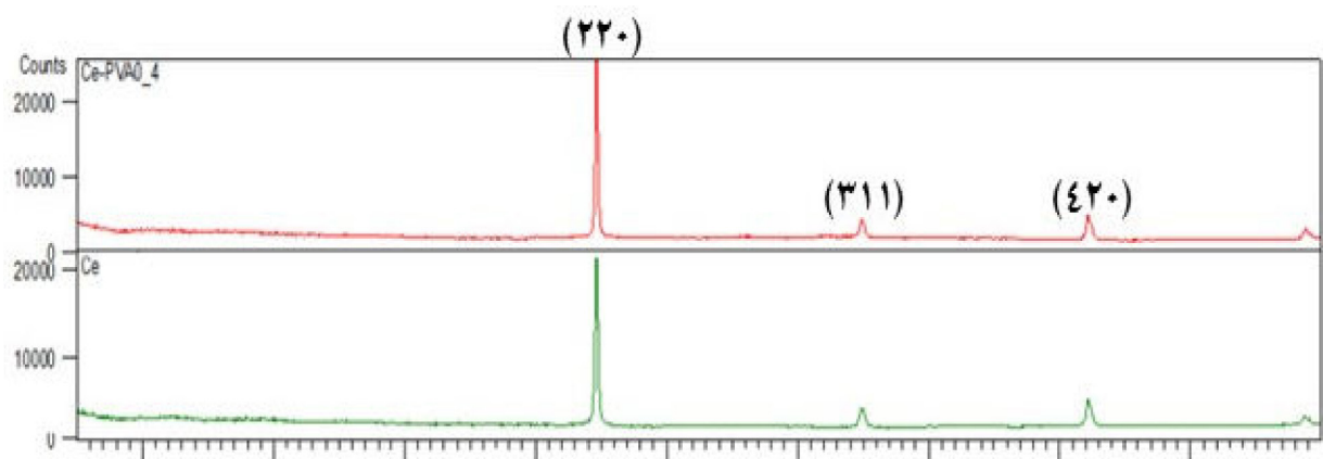
شکل ۶- نتایج آزمون XRD برای نمونه‌های پوشش داده شده در حمام پوشش تبدیلی پایه سربم در حضور PVA (بخش بالایی شکل) و در عدم حضور PVA (بخش پایینی شکل) در حمام.
