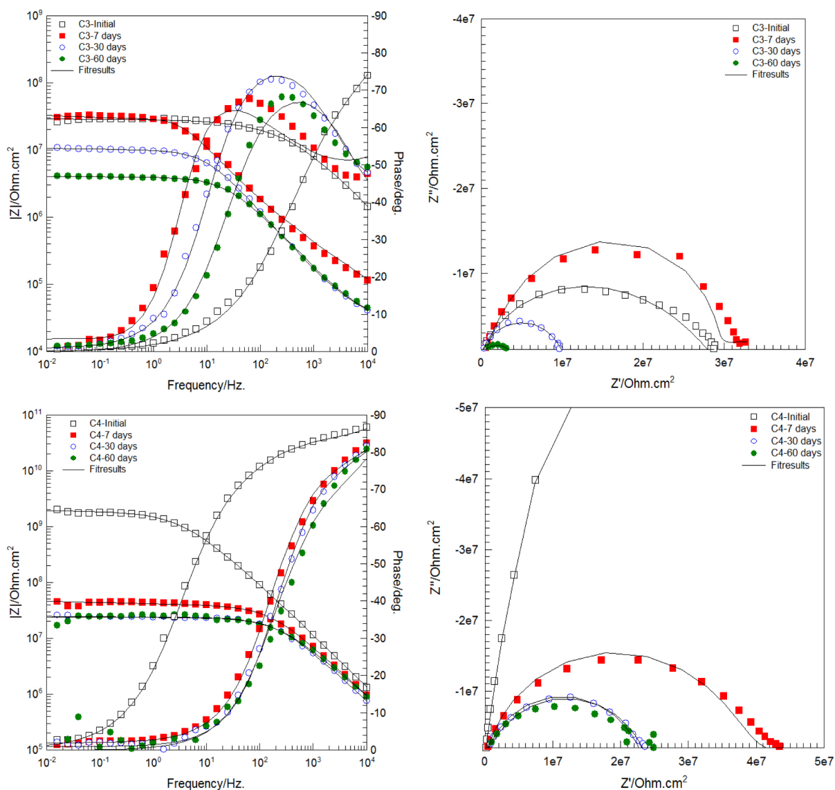
شکل ۷ - نمودارهای نایکوئیست و باد مربوط به نمونه پوشش‌های C3 (بالا) و C4 (پایین) طی زمان‌های مختلف غوطه‌وری در محلول کلرید سدیم ۳/۵ درصد.
