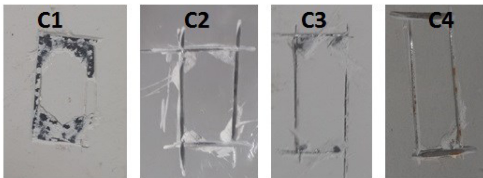
شکل ۴- نتایج چسبندگی پوشش‌های اپوکسی بعد از اتمام آزمایش خیساندن در آب 80^{\circ}\text{C} به مدت ۲۴ ساعت.
