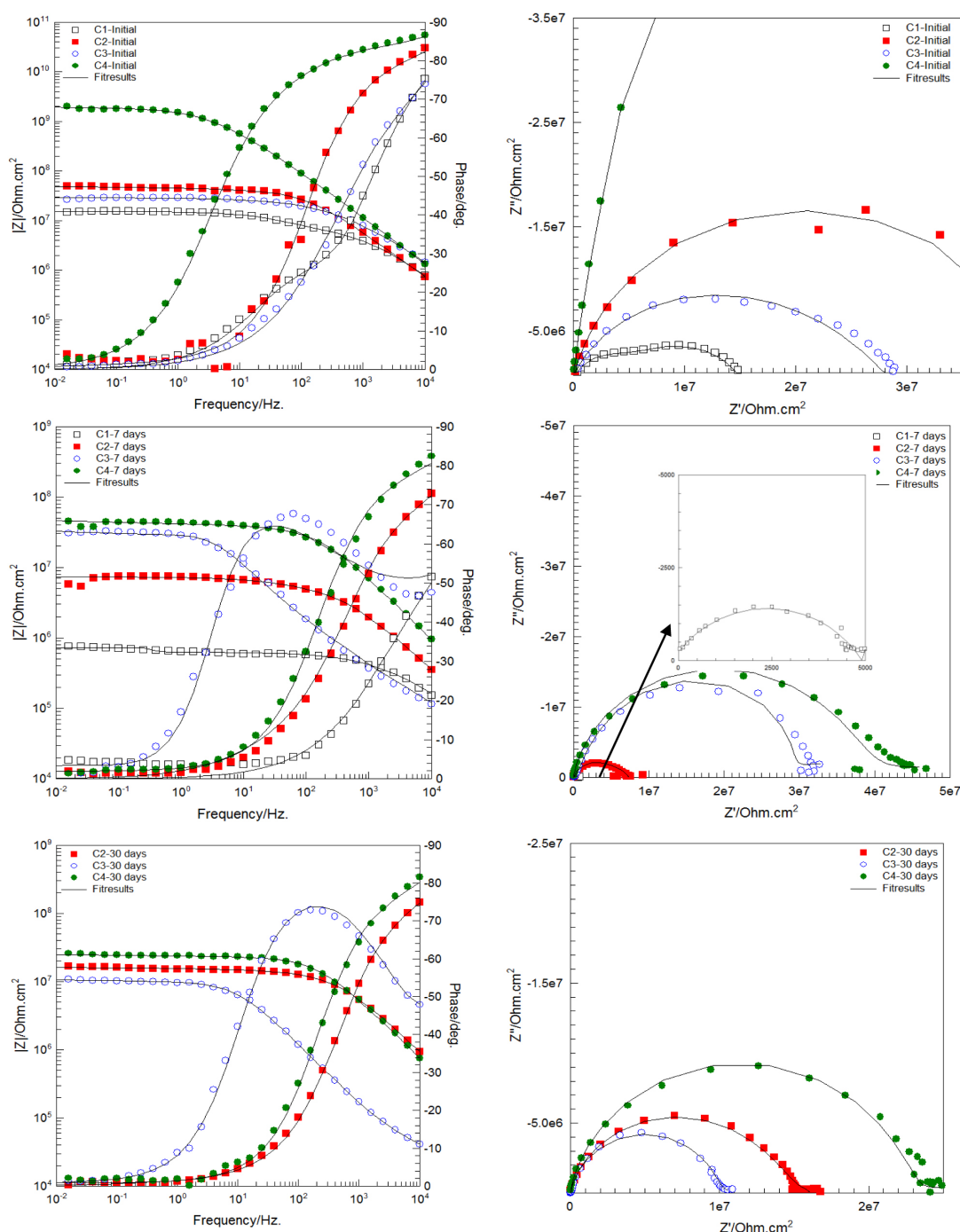
شکل ۶- نمودارهای نایکوئیست (راست) و باد (چپ) نمونه‌های مختلف در زمان‌های مختلف غوطه‌وری در محلول کلرید سدیم ۳/۵ درصد.
