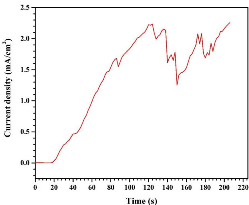
شکل ۱۱- منحنی پلاریزاسیون پتانسیواستاتیک برای محلول ۰/۱۸۷ M NaF + ۰/۰۶۳ M NaCl
