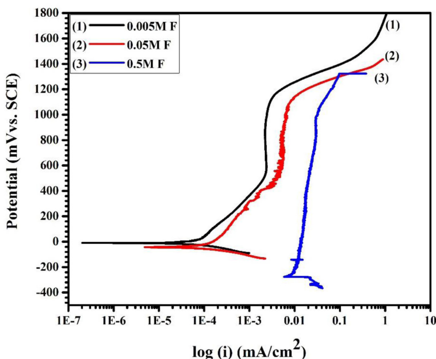
شکل ۴- منحنی پلاریزاسیون پتانسیو دینامیک برای سیم ارتودنسی NiTi در محلول فلوئوراید با غلظت‌های ۰/۰۰۵ و ۰/۰۵ و ۰/۵ مولار.
