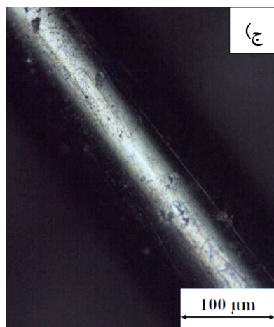
شکل ۱۲- حفرات تشکیل شده در سطح سیم ارتودنسی NiTi در محلول ۰/۰۵ مولار کلراید. الف) انتهای سیم در بزرگنمایی ۲۰۰ (ب) انتهای سیم در بزرگنمایی ۵۰۰ (ج) مرکز سیم در بزرگنمایی ۲۰۰ (د) مرکز سیم در بزرگنمایی ۵۰۰.
